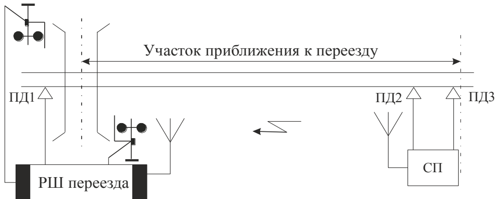
Рисунок 1 – Методы формирования и передачи информации о приближении поезда: а) дискретный; б) координатный.
