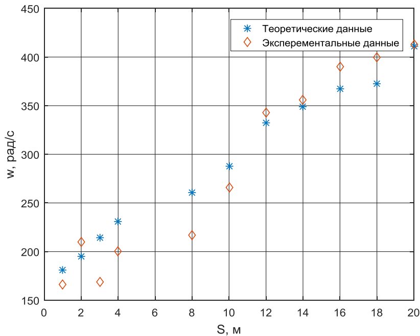
Рисунок 8 – Теоретические и экспериментальные данные зависимости пиковой частоты в АЧХ сигнала виброускорения от расстояния до точки приложения силы
