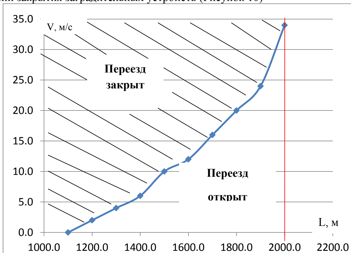
Рисунок 10 – График граничных значений скоростей от расстояний при t_{\text{и}} = \text{const} , для предлагаемой модели извещения
