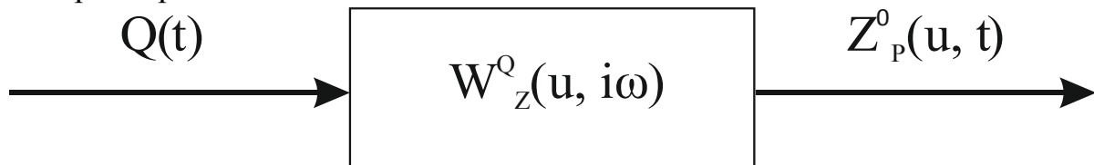
Рисунок 2 – Структурная схема преобразования силы в точке контакта колеса и рельса
